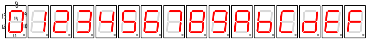
Figura 5. Representação dos dígitos de 0 a F no display de 7 segmentos.
